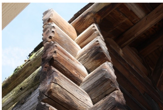
Blockbau Obergeschoss
